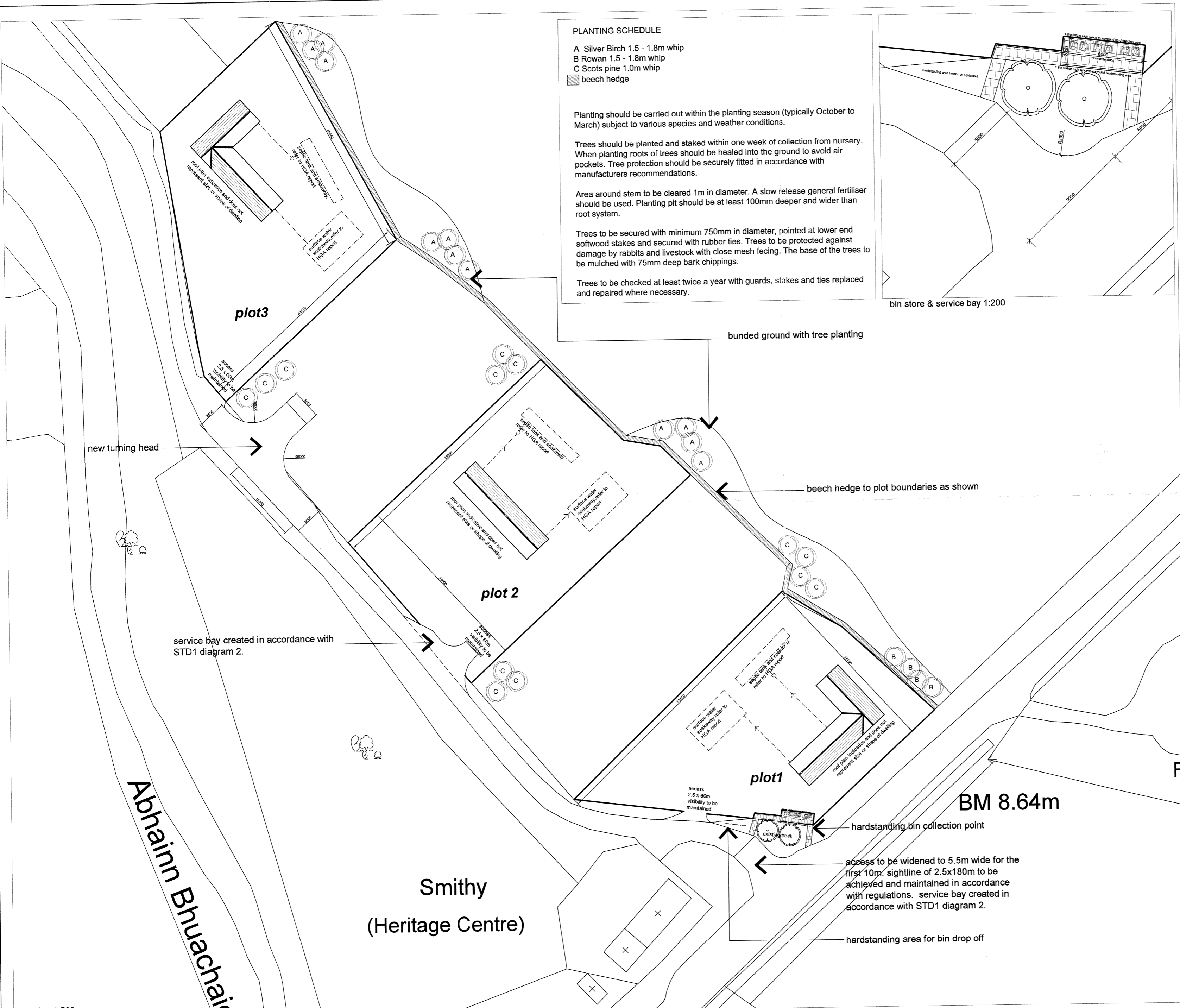
site plan 1:500
